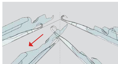
Schiebernadel mit speziellem Schieber für die Umhängfunktion
